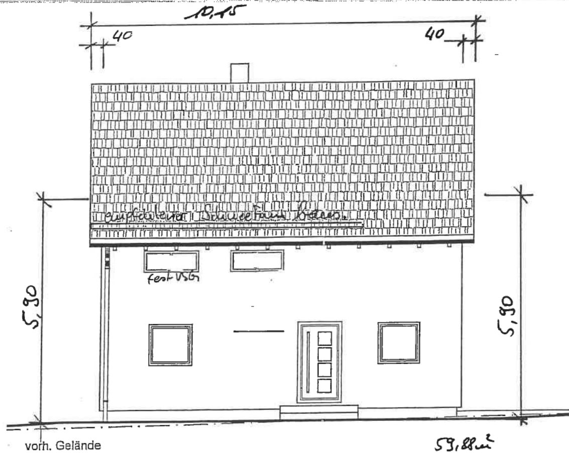
Ansicht Westen
