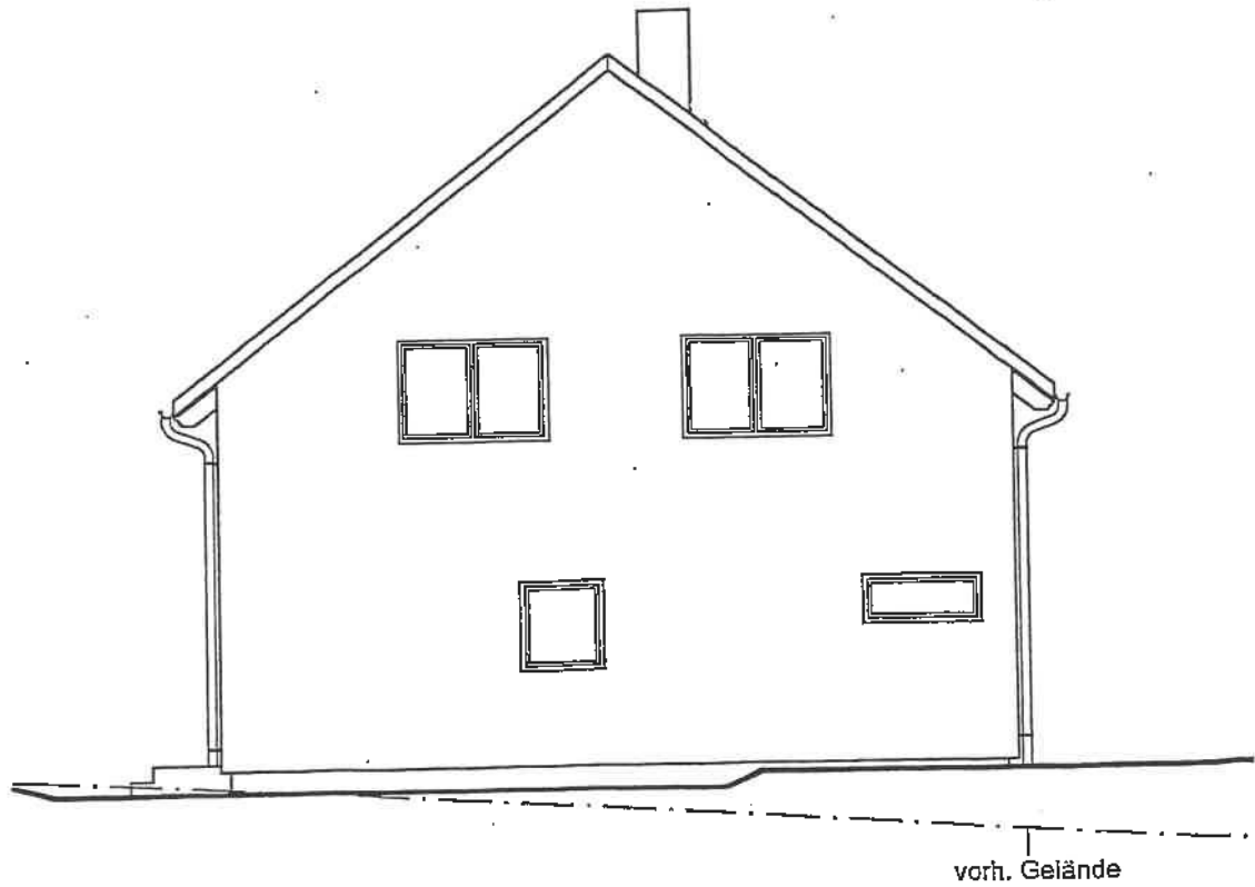
Ansicht Süden
