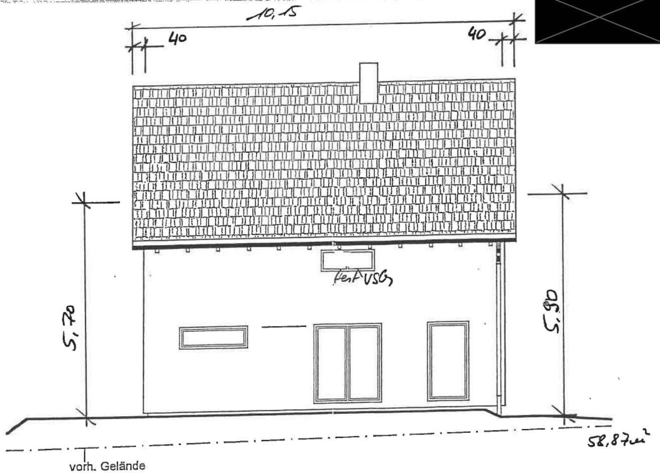
Ansicht Osten
