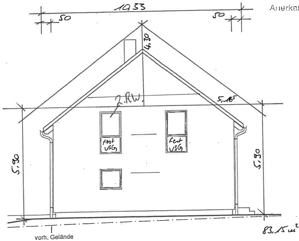
Ansicht Norden
