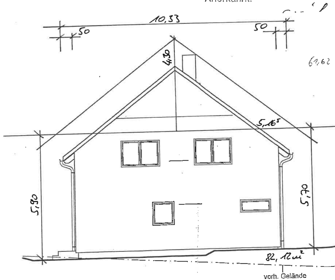
Ansicht Süden
